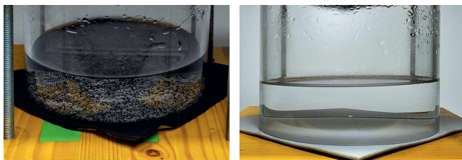
Abb. 1: Elution von der Prüfkörperoberfläche mit deionisiertem Wasser; links: EPDM, rechts: FPO
