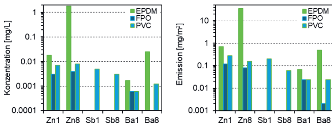
Abb. 3: Konzentrationen (links) und freigesetzte Emissionen (rechts) der nachweisbaren Elemente Zink (Zn), Antimon (Sb) und Barium (Ba) in der Mischprobe (1) und Eluat 8 für drei Kunststoffdichtungsbahnen
