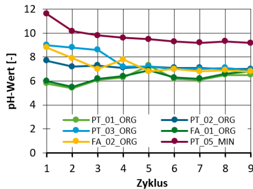
Abbildung 58: pH-Werte der untersuchen vier Putze und zwei Farben
