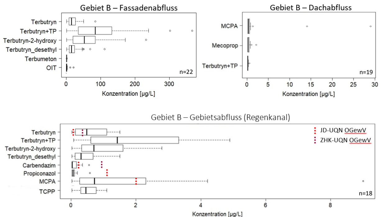
Abbildung 20: Spurenstoff-Konzentrationen in Fassaden-, Dach- und Gebietsabfluss von Gebiet B
