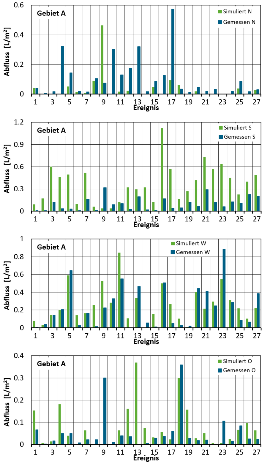
Abbildung 68: Vergleich Fassadenabfluss simuliert und gemessen für die Nord-, Süd-, West- und Ostfassade in Gebiet A
