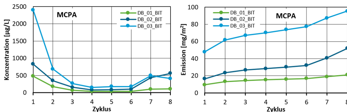
Abbildung 32: Konzentrationen und kumulierte Emissionen von MCPA in den drei untersuchten Bitumenbahnen (wurzelfest: DB_02 und DB_03)
