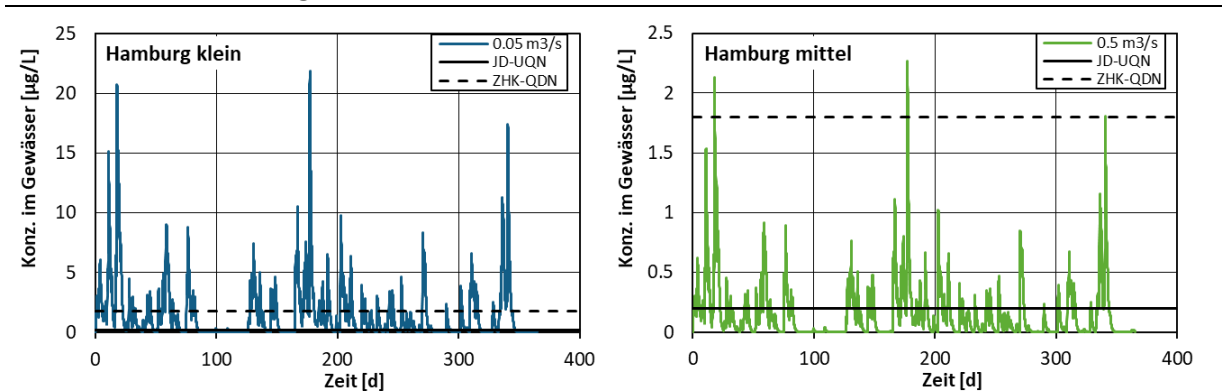
Abbildung 41: Konzentrationen von Diuron im kleinen (links) und mittleren Gewässer (rechts) von Hamburg
