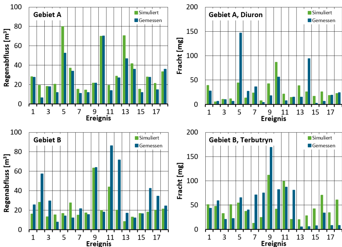
Abbildung 37: Regenabfluss (links) und Emissionen (rechts) der in den Regenkanal entwässernden Flächen von Gebiet A (oben) und Gebiet B (unten).
