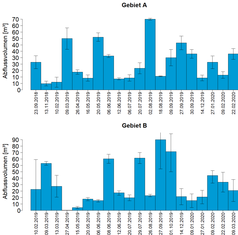
Abbildung 51: Abflussvolumen der analysierten Regenereignisse im Regenkanal für Gebiet A und B
