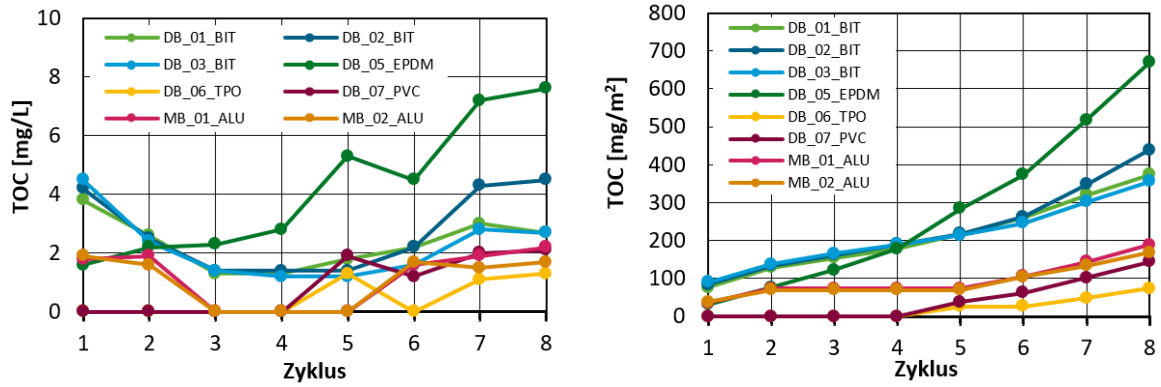
Abbildung 67: Konzentration und kumulierte TOC Emission der acht im DSLT eluierten Bauprodukte
