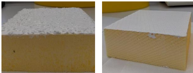
Abbildung 28: Prüfkörper beschichtet mit Putz (links) und doppeltem Farbanstrich (rechts)
