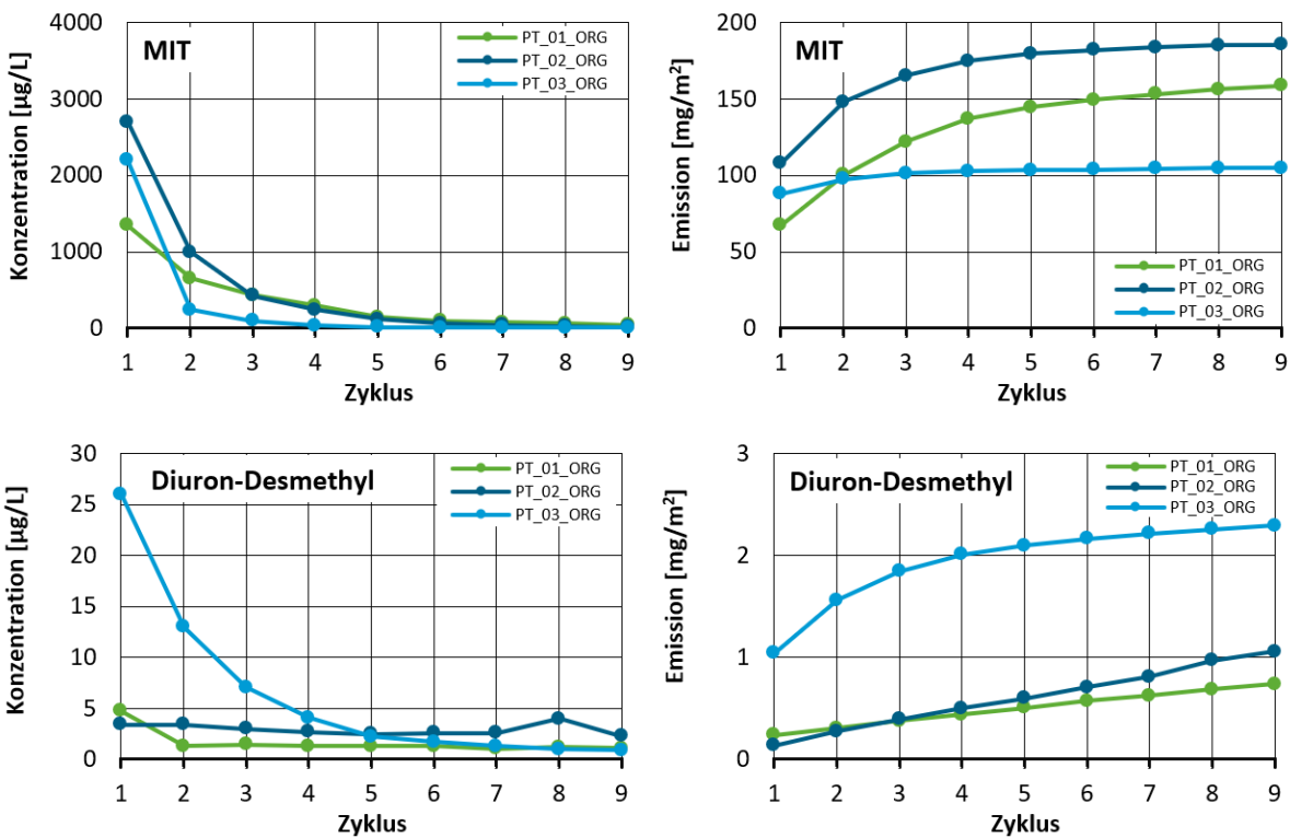
Abbildung 61: Konzentrationen und kumulierte Emissionen von MIT (oben) und Diuron-Desmethyl (unten) in drei Putzen
