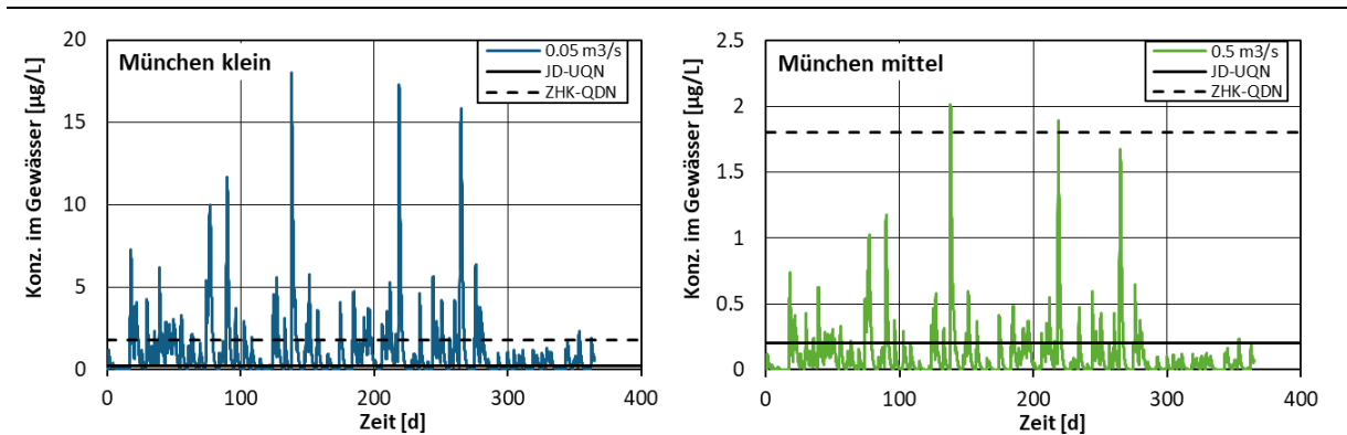
Abbildung 73: Diuron-Konzentrationen im kleinen (links) und mittleren Gewässer (rechts) für München.
