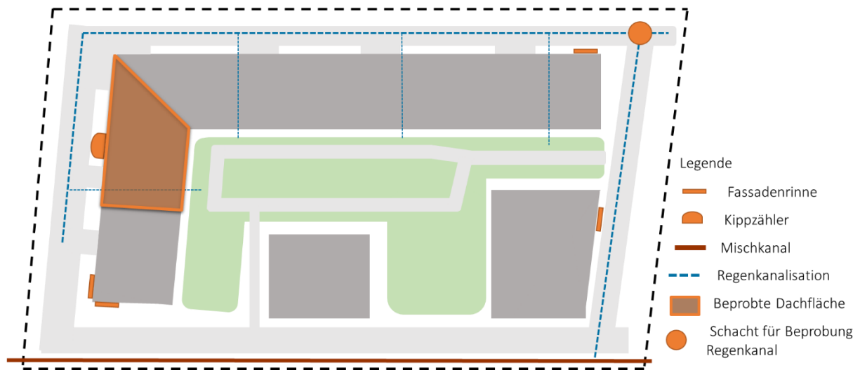
Abbildung 5: Regenentwässerung von Testgebiet B
