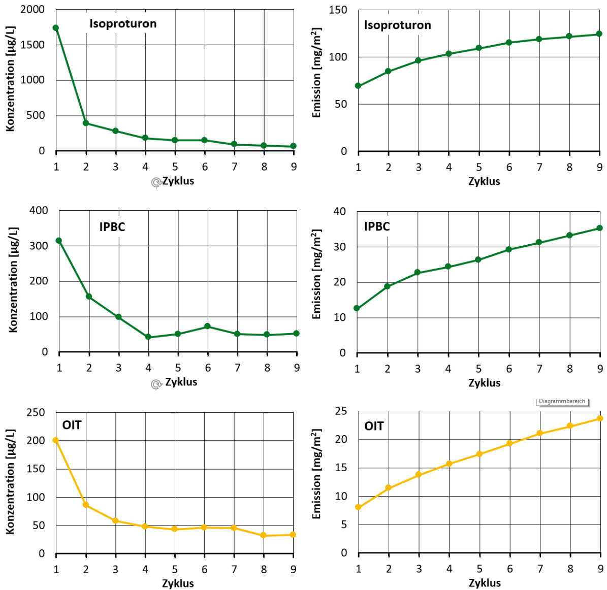
Abbildung 63: Konzentration und kumulierte Emission von Isoproturon (oben), IPBC (Mitte) in der Farbe Gebiet A (FA_01_ORG) und OIT (unten) in der Farbe von Gebiet B (FA_02_ORG)
