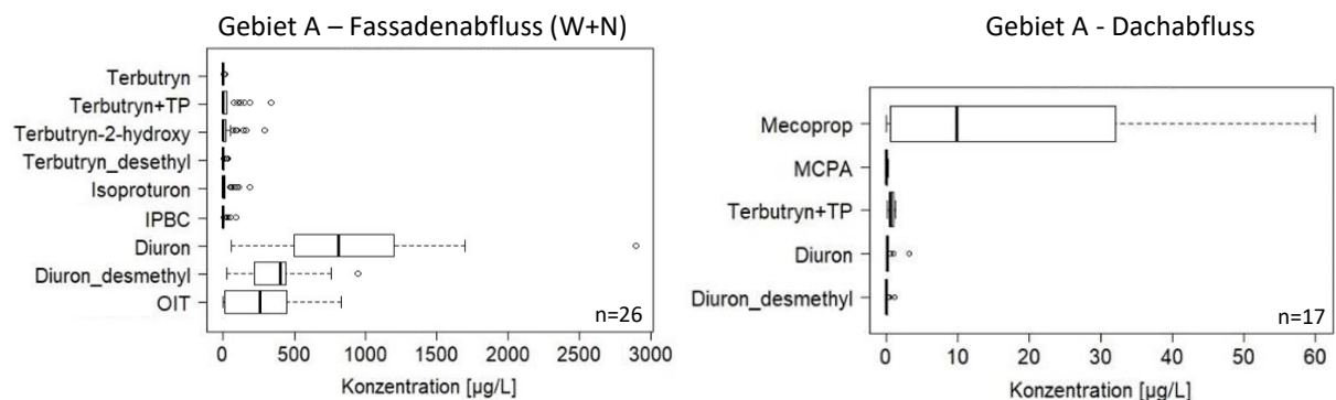
Abbildung 15: Spurenstoff-Konzentrationen in Fassaden- und Dachabfluss von Gebiet A
