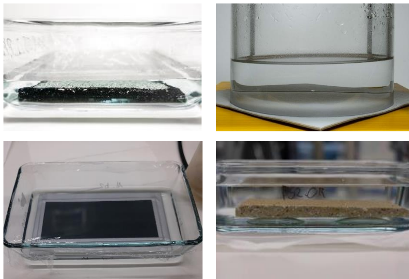
Abbildung 29: Prüfkörper im DSLT: Bitumenbahn (links oben), PE-beschichtetes Metallblech (links unten), FPO-Kunststoffdichtungsbahn (rechts oben) und Pflasterstein (rechts unten)
