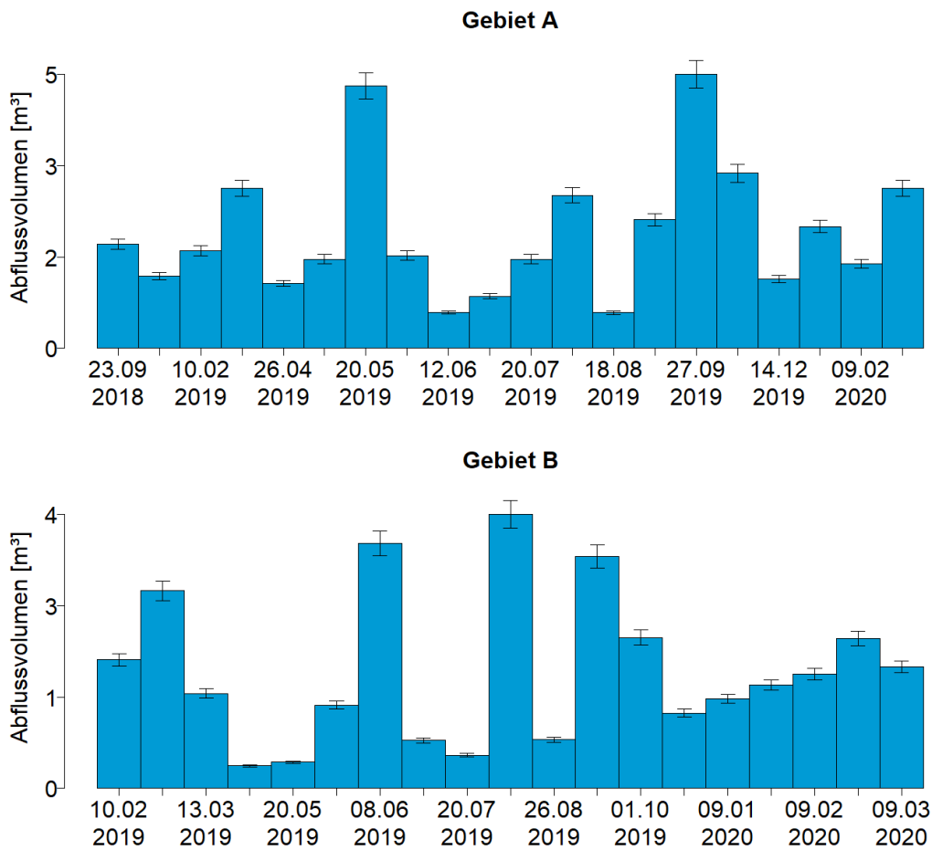
Abbildung 52: Abflussvolumen der analysierten Regenereignisse im Dachablauf für Gebiet A und B
