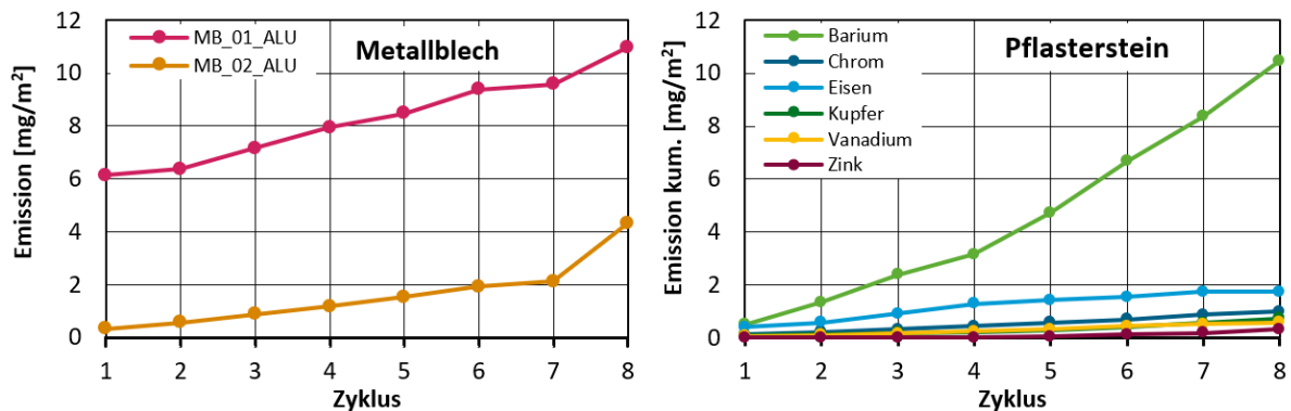
Abbildung 33: Kumulierte Emissionen von Aluminium aus Alublechen (links) und sechs Elementen aus einem Pflasterstein (rechts)
