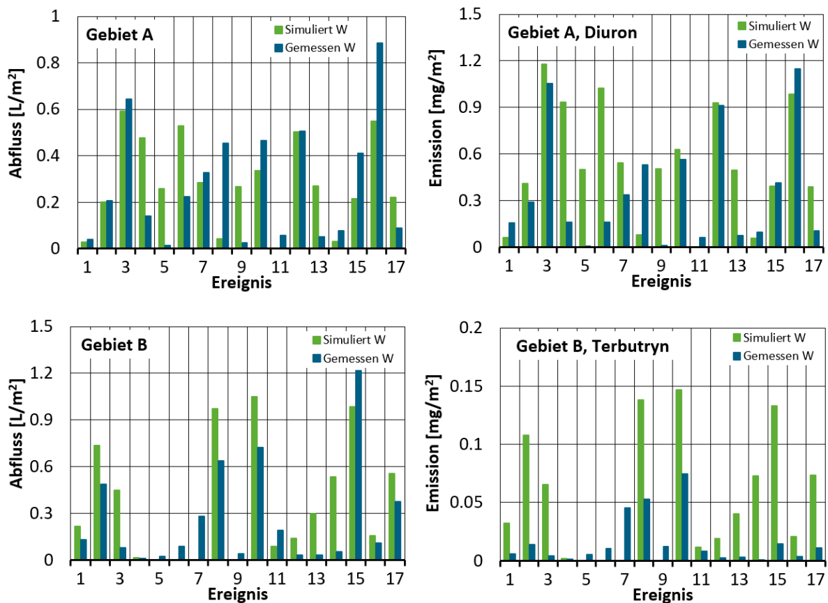
Abbildung 36: Fassadenabfluss und Fracht der ereignisbezogenen Diuron-Fracht an der Westfassade von Gebiet A (oben) und der Terbutryn-Fracht von Gebiet B (unten)
