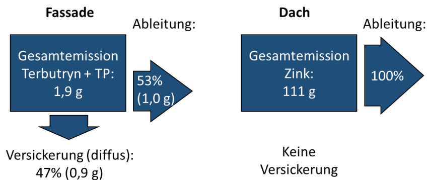
Abbildung 26: Stoffbilanz für den Regenkanal und diffuses Versickern für die Emissionen aus Fassade und Dach für Terbutryn und Transformationsprodukte sowie Zink in Gebiet B
