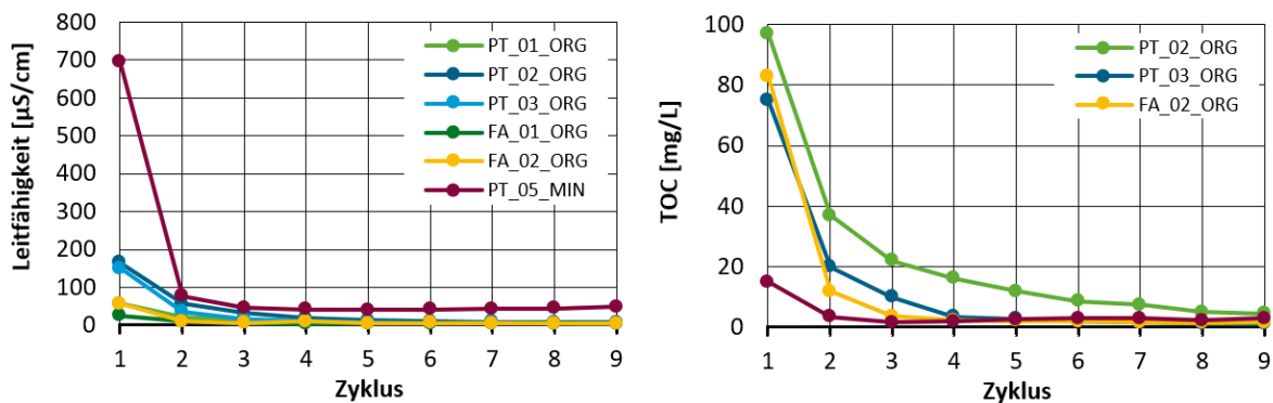
Abbildung 59: Elektrische Leitfähigkeit (links) und gesamter organischer Kohlenstoff (TOC; rechts) der untersuchen Putze und Farben
