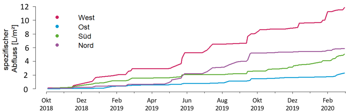
Abbildung 48: Kumulierter spezifischer Abfluss der Fassaden für Gebiet B
