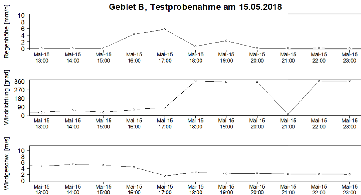
Abbildung 44: Hydrometeorologische Verhältnisse bei der Testprobenahme am 15.05.2018 im Testgebiet B.
