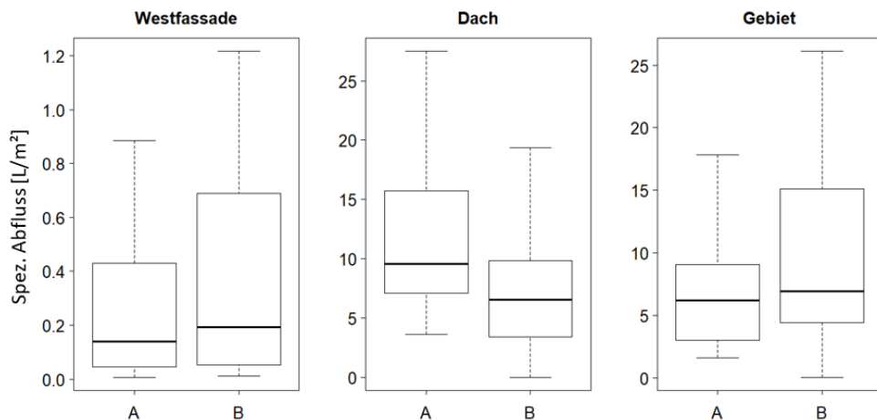
Abbildung 14: Spezifische Abflussmenge der analysierten Regenereignisse für Gebiet A und B (n=20)
