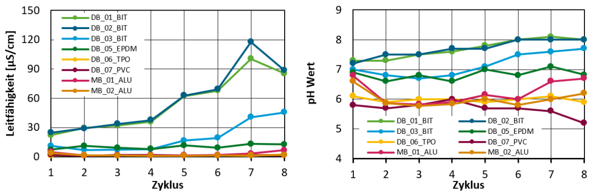
Abbildung 66: Elektrische Leitfähigkeit und pH-Werte in Eluaten der Bauprodukte
