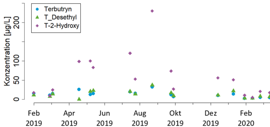
Abbildung 21: Konzentrationsverlauf für Terbutryn und die Transformationsprodukte Desethyl-Terbutryn und Hydroxy-Terbutryn im Fassadenabfluss der Westfassade in Gebiet B
