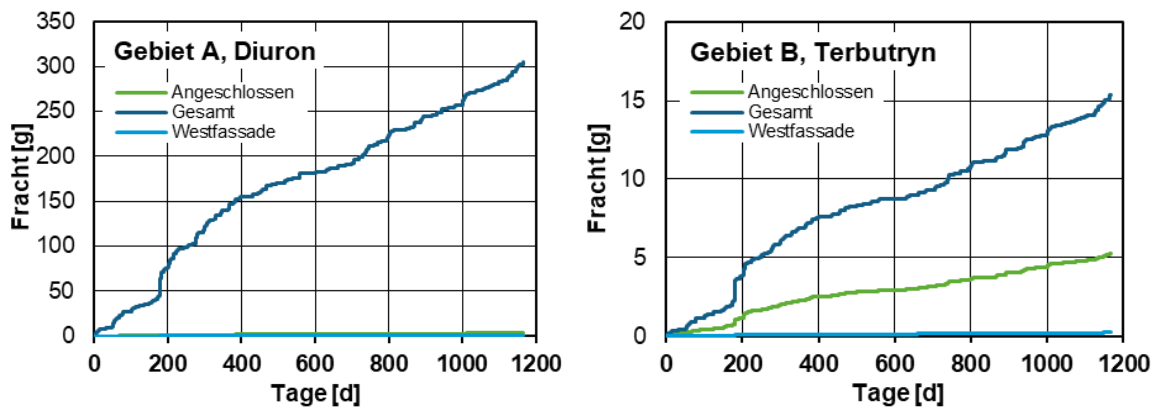
Abbildung 71: Modellierte Frachten für die beprobte Westfassade, die an den Regenkanal angeschlossenen Fassaden sowie die Gesamtfrachten für Gebiet A (links) und Gebiet B (rechts)
