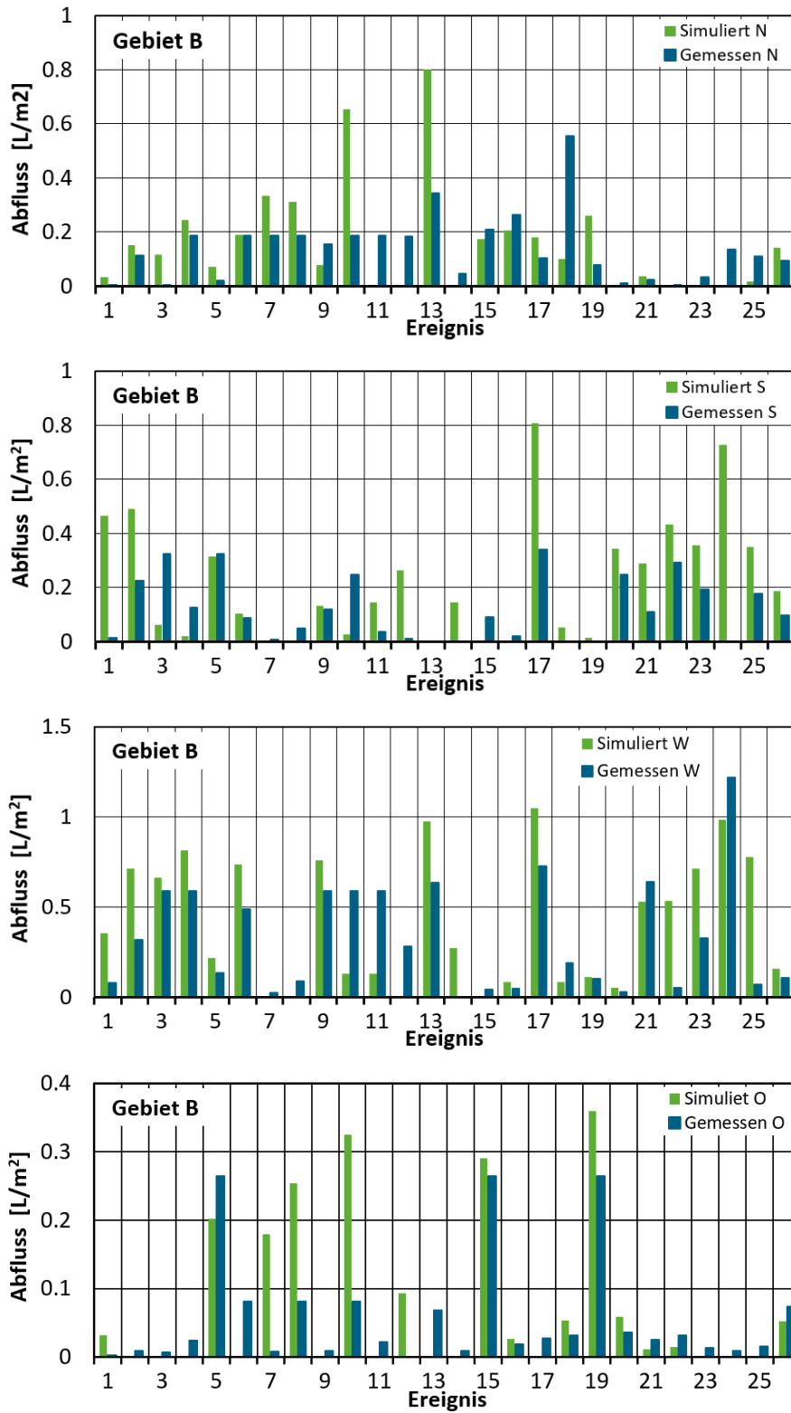
Abbildung 69: Vergleich Fassadenabfluss simuliert und gemessen für die Nord-, Süd-, West- und Ostfassade in Gebiet B
