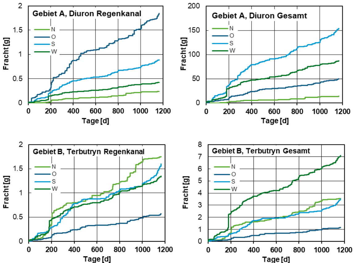
Abbildung 38: Expositionsabhängige Biozidemissionen der Fassaden in den Regenkanal (=angeschlossen, links) und expositionsabhängige Gesamtemissionen aller Gebädefassaden (rechts) von Gebiet A (oben) und Gebiet B (unten).
