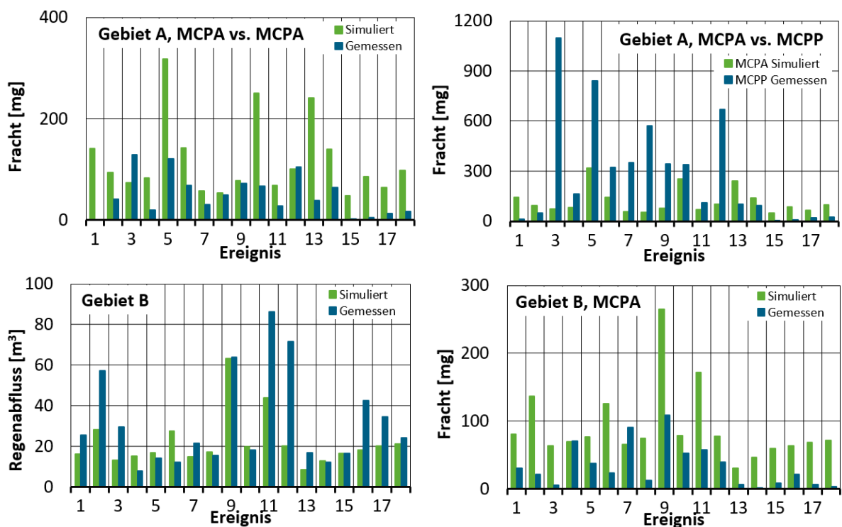
Abbildung 75: Simulierte und gemessene MCPA-Fracht (oben links) und gemessene MCPP-Fracht (oben rechts) für Gebiet A, Vergleich von Abfluss (unten links) und MCPA-Emission (unten rechts) der angeschlossenen Flächen von Gebiet B.
