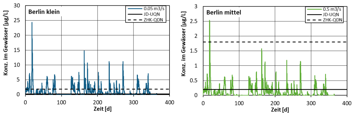
Abbildung 72: Diuron-Konzentrationen im kleinen (links) und mittleren Gewässer (rechts) für Berlin.
