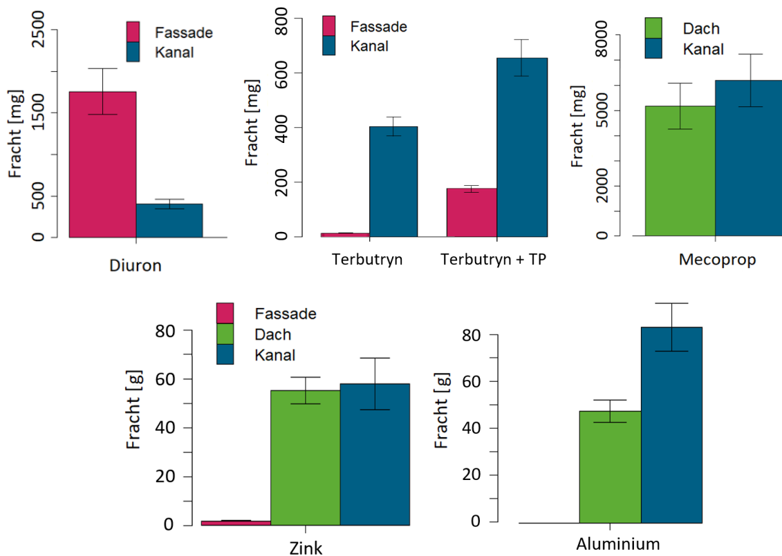
Abbildung 23: Frachten in Fassaden-, Dach- und Gebietsabfluss für ausgewählte Stoffe in Gebiet A
