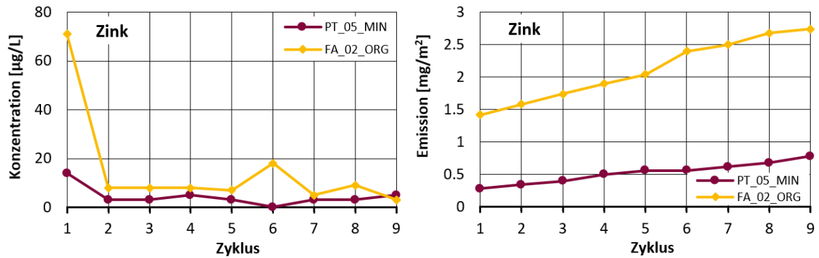
Abbildung 64: Konzentration und kumulierte Emission von Zink aus mineralischem Putz und der Farbe von Gebiet B (FA_02_ORG)
