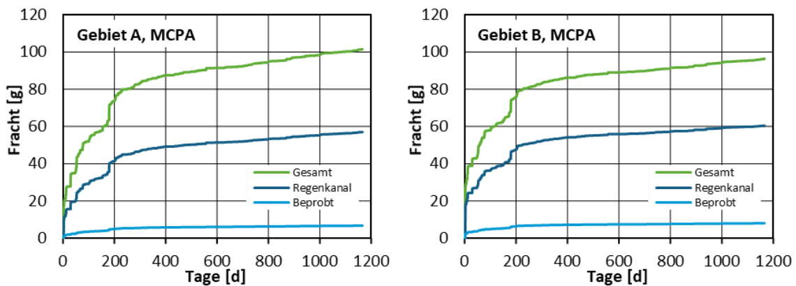
Abbildung 76: Emissionen der beprobten Dachflächen, der in den Regenkanal entwässernden Dächern und für der Dachflächen des Gesamtgebiet in Gebiet A (links) und Gebiet B (rechts)
