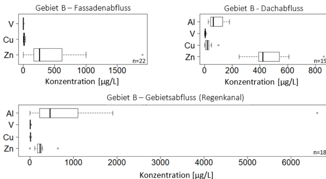
Abbildung 22: Schwermetall-Konzentrationen in Fassaden-, Dach- und Gebietsabfluss in Gebiet B
