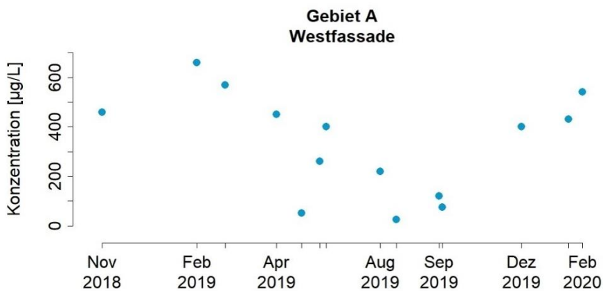
Abbildung 53: Konzentrationsverlauf von OIT im Fassadenablauf (West) in Gebiet A
