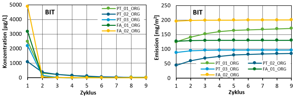
Abbildung 60: Konzentrationen und kumulierte Emissionen von BIT in drei organischen Putzen aus Gebiet A und zwei Farben der Gebiete A und B
