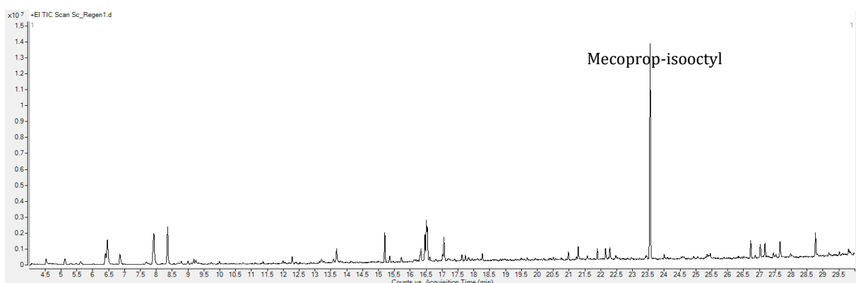
Abbildung 45: GC-Chromatogramm Regenablauf 1
