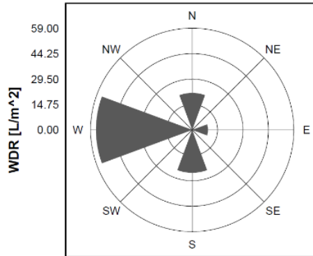
Abbildung 70: Schlagregensmengen differenziert nach Windrichtung im Gebiet B
