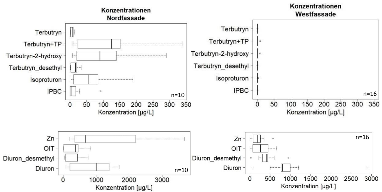
Abbildung 18: Konzentrationen in Fassadenabfluss der West- und Nordfassade in Gebiet A
