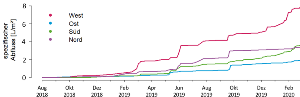
Abbildung 13: Gemessener, kumulierter spezifischer Abfluss der Fassaden für Gebiet A
