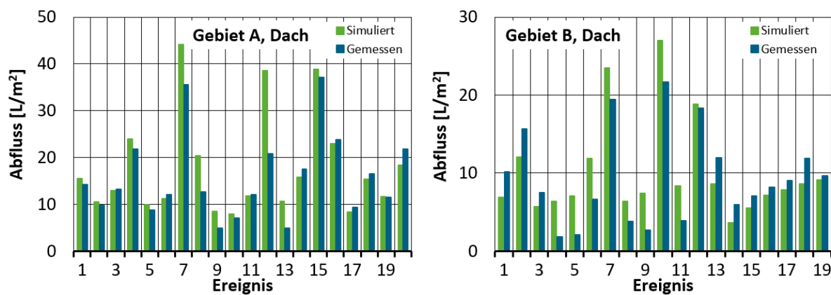
Abbildung 35: Dachabfluss simuliert und gemessen für die beprobten Dachflächen von Gebiet A (links) und Gebiet B (rechts).
