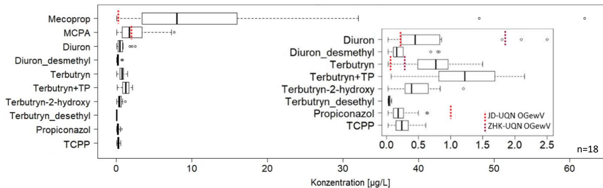
Abbildung 16: Spurenstoff-Konzentrationen im Gebietsabfluss (Regenkanal) von Gebiet A
