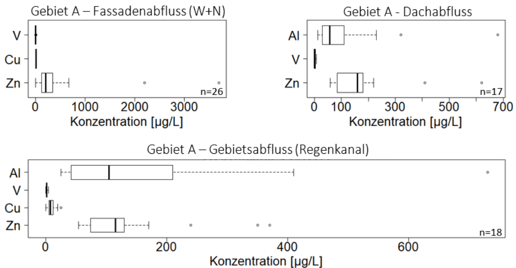
Abbildung 19: Schwermetall-Konzentrationen in Fassaden-, Dach- und Gebietsabfluss in Gebiet A
