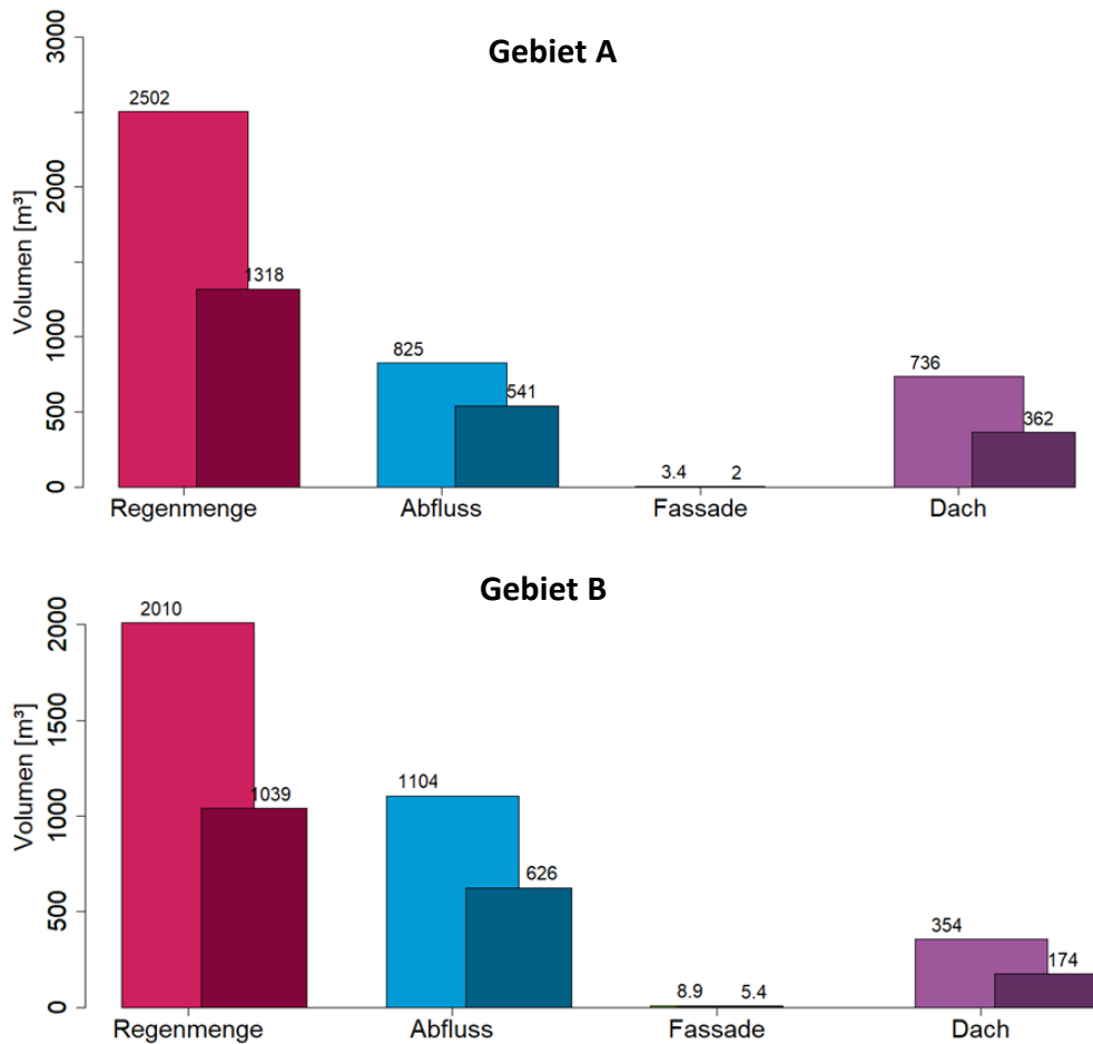
Abbildung 12: Volumina der Regenmenge und der in den Regenkanal entwässernden Dach-, Fassaden- und Gebietsabflüsse für Gebiet A und B. Hell: erfasste Regenereignisse; dunkel: analysierte Regenereignisse
