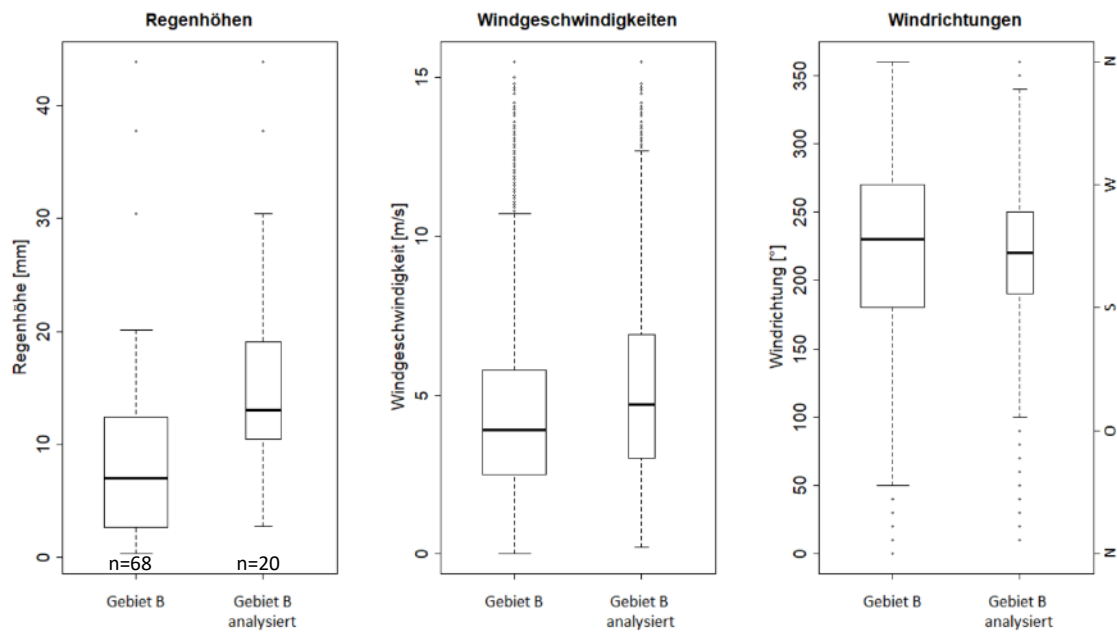
Abbildung 50: Regenhöhe und Winddaten für erfasste und analysierte Regenereignisse in Gebiet B
