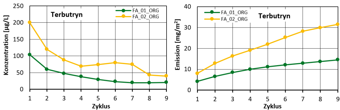
Abbildung 31: Konzentrationen und kumulierte Emissionen von Terbutryn in den beiden Farben von Gebiet A (FA_01_ORG) und Gebiet B (FA_02_ORG).
