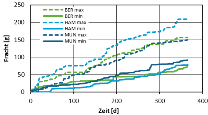
Abbildung 39: Kumulierte Stofffracht bei minimalem und maximalem Jahresniederschlag (min, max) an den Standorten Berlin, Hamburg und München.
