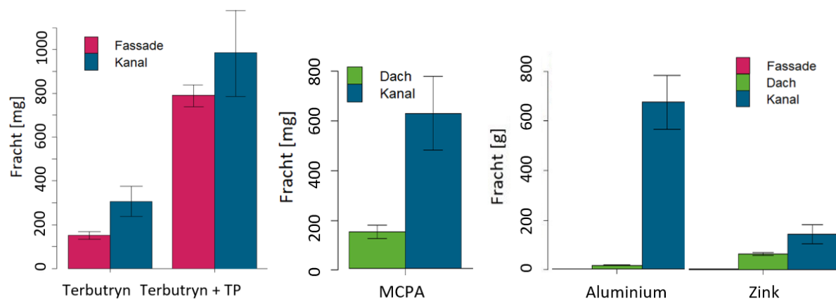
Abbildung 25: Frachten in Fassaden-, Dach- und Gebietsabfluss für ausgewählte Stoffe in Gebiet B
