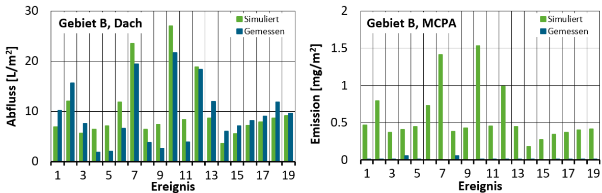
Abbildung 74: Dachabfluss und ereignisbezogene MCPA-Fracht am beprobten Dach von Gebiet B
