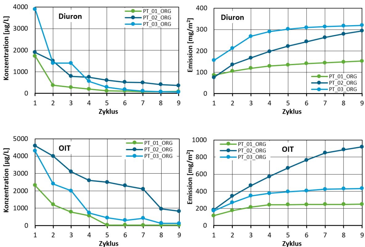
Abbildung 30: Konzentrationen und kumulierte Emission von Diuron (oben) und OIT (unten) in den drei Putzen von Untersuchungsgebiet A
