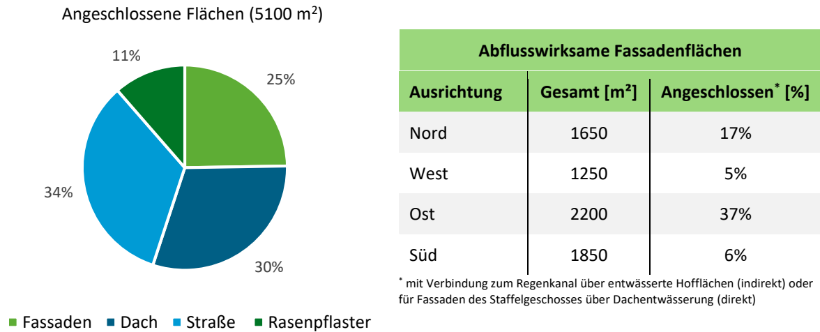
Abbildung 3: Flächenübersicht für Testgebiet A. Anteile der in den Regenkanal entwässernden Flächen (links) und abflusswirksame Fassadenflächen nach Ausrichtung (rechts)
