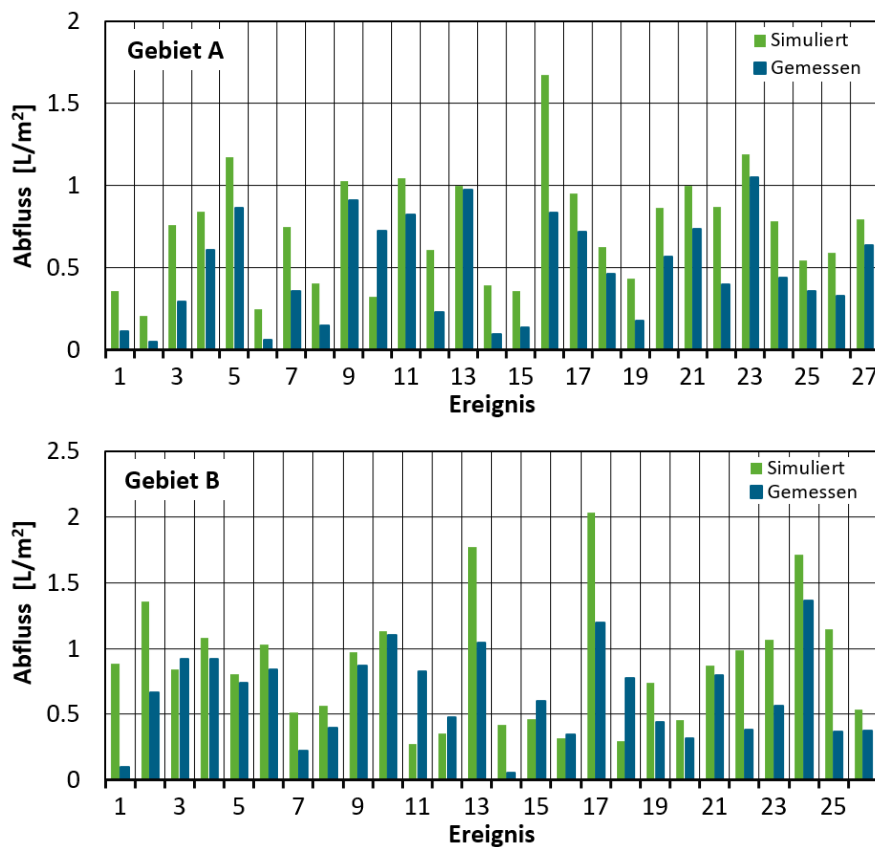
Abbildung 34: Fassadenablauf simuliert und gemessen für alle Fassaden des Gebietes A (oben) und B (unten). Berücksichtigt sind Ereignisse \geq 10 mm Niederschlag.
